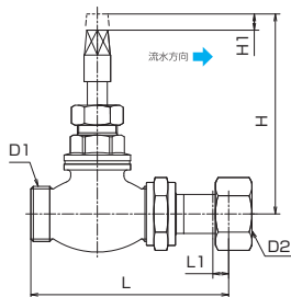
●主要部寸法表
