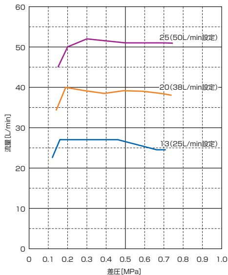
■ 定流量弁の流量特性
