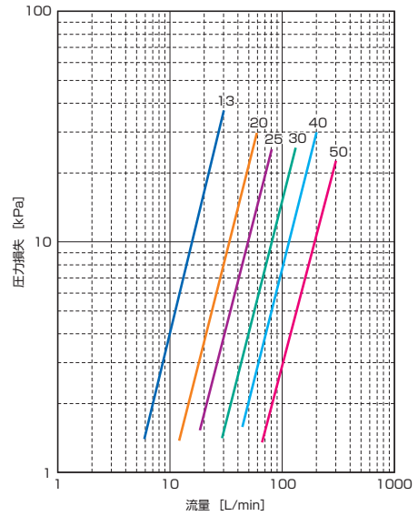
■ 平行おねじ(甲)の圧力損失
