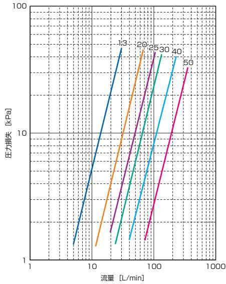
■ 平行おねじ・伸縮の圧力損失
