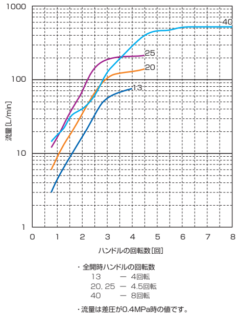
■ アクスバルブの開度による流量特性
